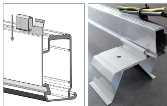
Exemples d'accessoires compatibles avec le CLIPS'OBAC (crochets chemin de câbles, mise à la terre...)
