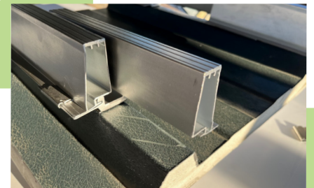
Fixation des rails par S-CLIP
